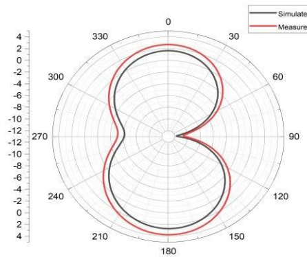
Fig 17. Result of E-plane. 2.4 GHz
