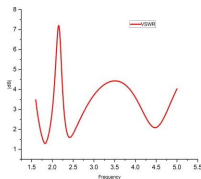
Fig.4. VSWR
